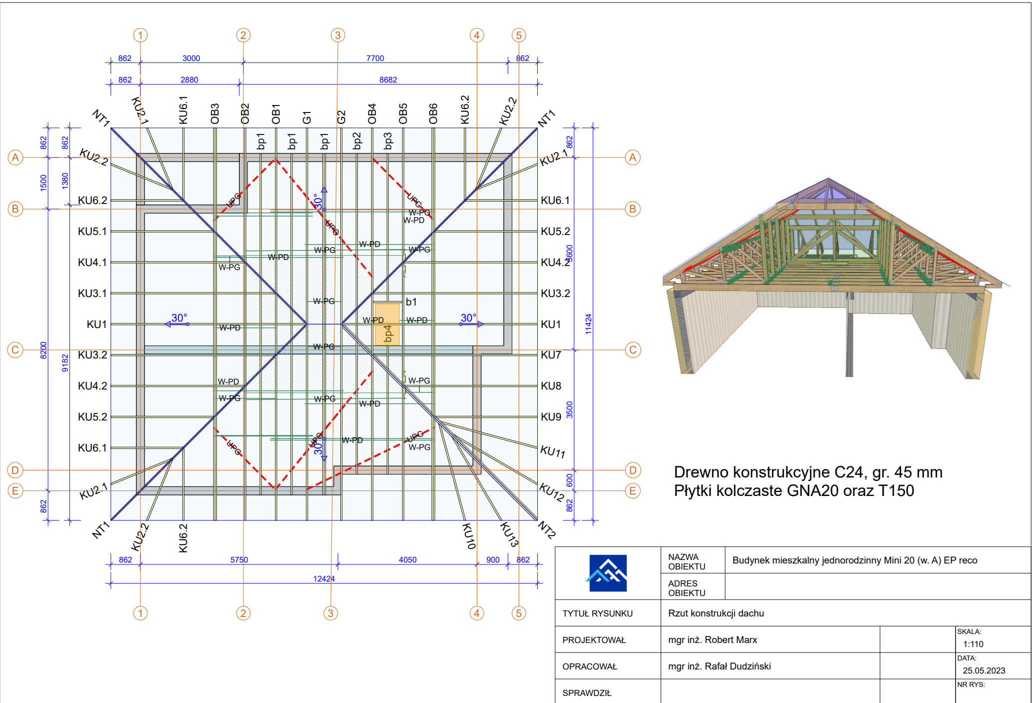
Prefabrykowana więźba dachowa - dom parterowy Mini 20 (w. A) EP reco
