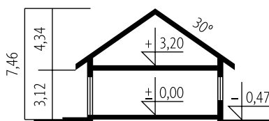
Schemat przekroju
